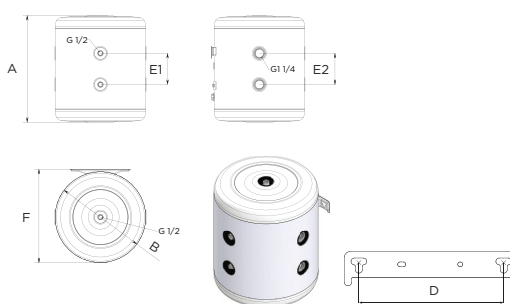
BF100 - Medidas
