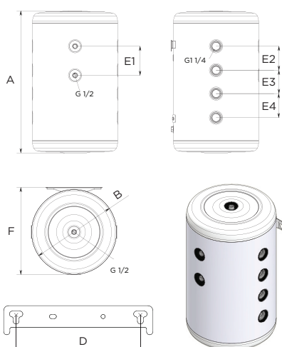
BF080 - Medidas
