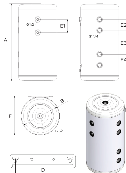
BF100 - Medidas
